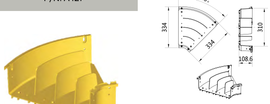
45° Horizontal Curve P/N: A427
