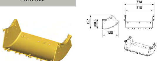
45° Up Curve P/N: A406
