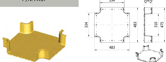
Horizontal Cross P/N: A407
