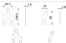
Kit coupler spill over P/N: T2043
