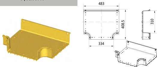
Horizontal T P/N: A417
