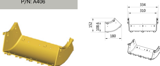
45° Up Curve P/N: A406
