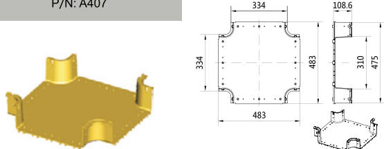
Horizontal Cross P/N: A407
