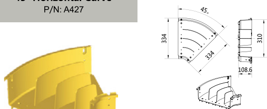
45° Horizontal Curve P/N: A427
